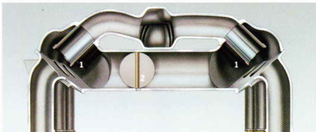
Varioram. Système d'admission à résonance: rallonge de collecteur (1) et clapets de résonance (2) ouverts. Davantage de puissance à régime élevé.
