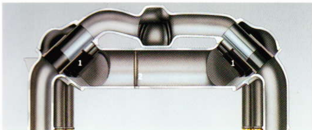
Varioram. Système d'admission monochambre: rallonge de collecteur (1) et clapets de résonance (2) fermés. Davantage de couple à faible et moyen régimes.
